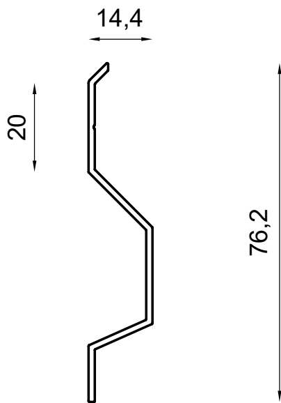
Listwa cokołowa - dociskowa C1
